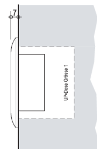
Seitenansicht (Maß: 1:3)
